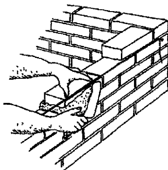
Figura 8 - Retirada do excesso de argamassa
