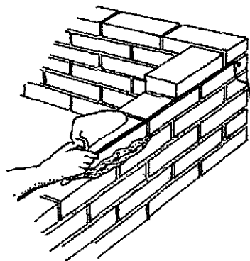
Figura 7 - Assentamento do tijolo
